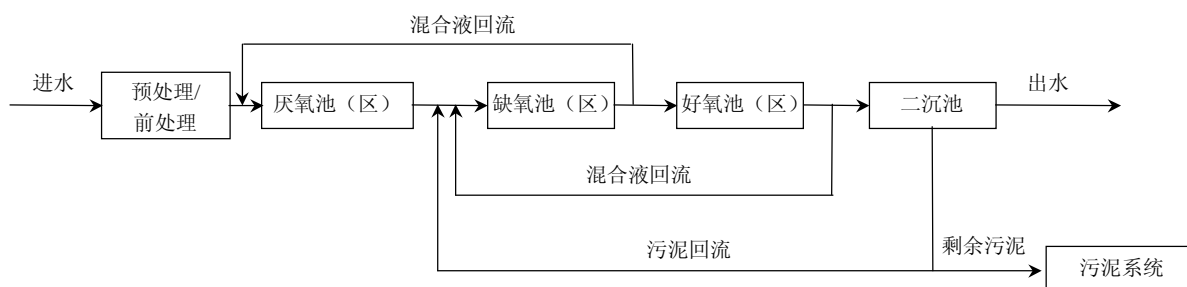
图 A.1 UCT 工艺流程图
