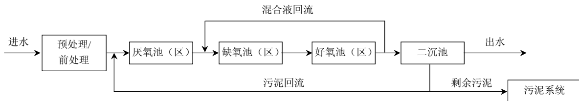
图 3 厌氧缺氧好氧工艺流程图
