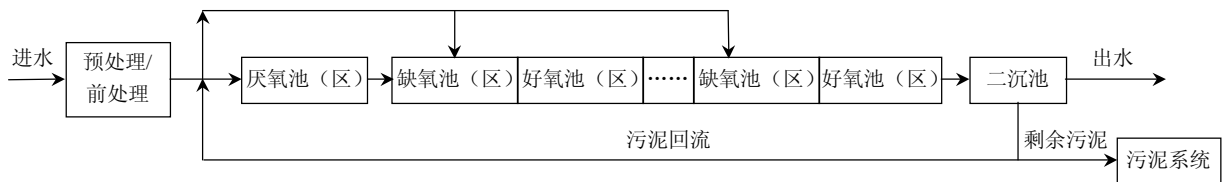
图 A.5 MAO 工艺流程图
